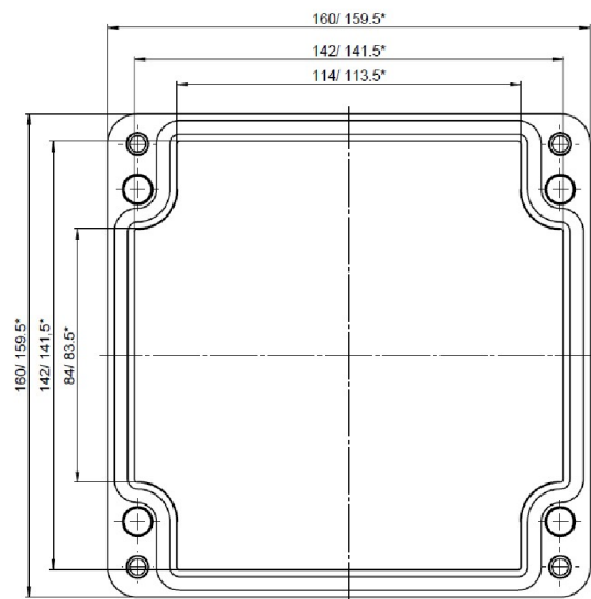
Deckel / Lid
